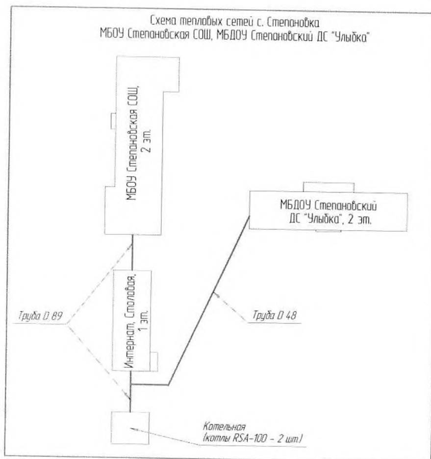
Рисунок 4.2 – Схема теплоснабжения МБОУ Степановская СОШ, МБДОУ Степановский ДС «Улыбка»
