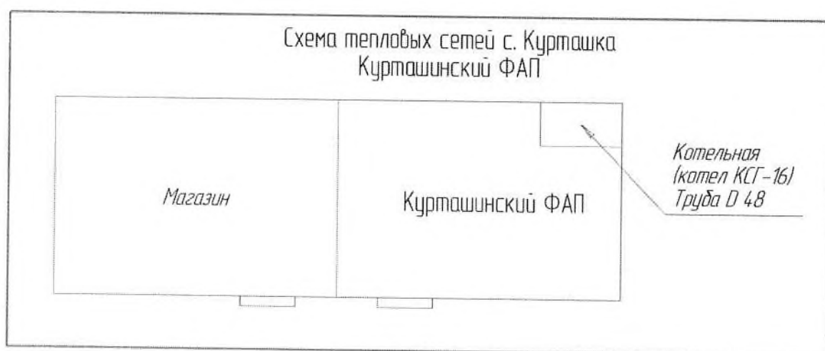
Рисунок 4.7 – Схема теплоснабжения Курташинский ФАП
