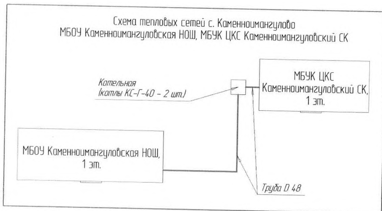
Рисунок 4.9 – Схема теплоснабжения МБОУ Каменноимангуловская НОШ, МБУК ЦКС Каменноимангуловский СК
